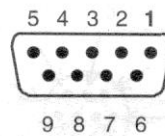
DB9 femelle
